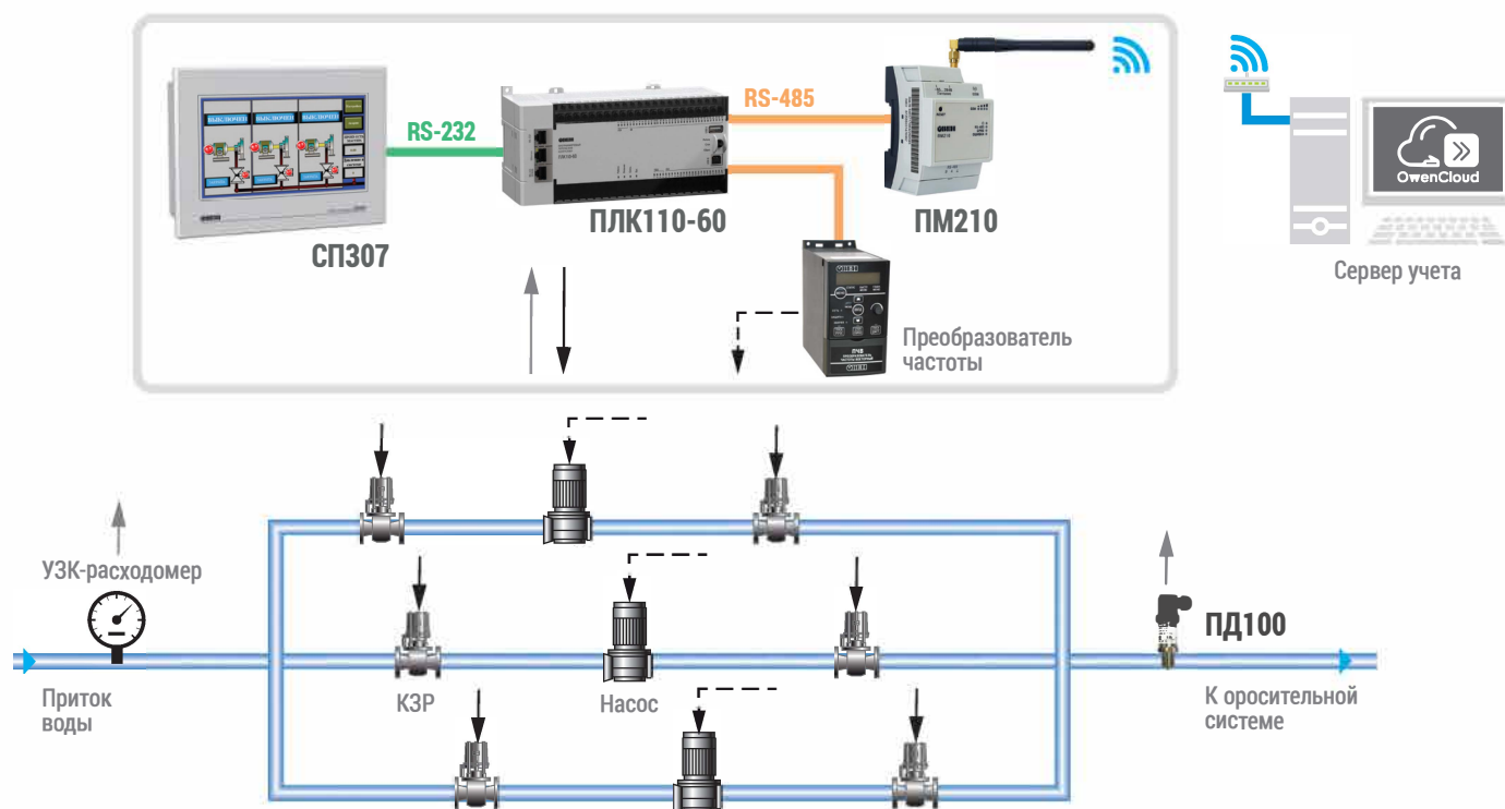
Функциональная схема управления насосной станцией
