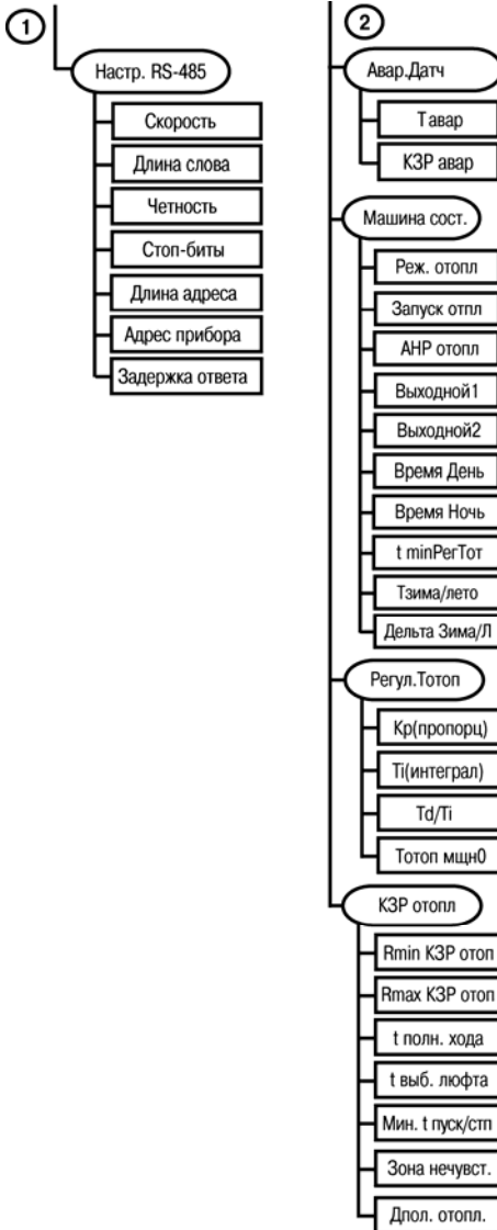
Рисунок И.1 – Главное меню прибора (продолжение)
