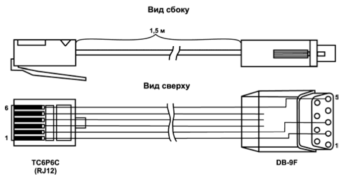
Рисунок Д.2 – Схема кабеля КС2
