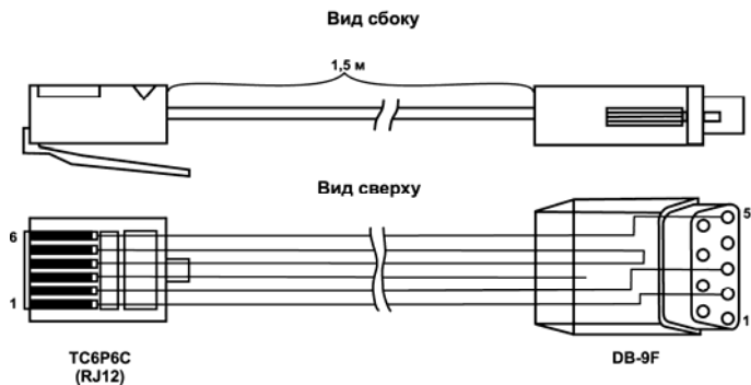
Рисунок Д.1 – Схема кабеля КС1
